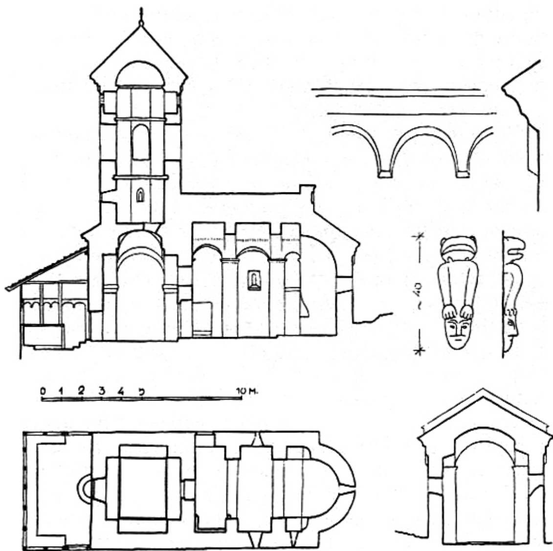
Скица храма, основа, пресеци и детаљи
